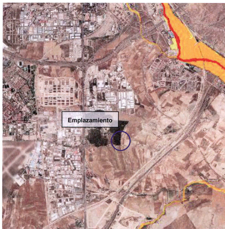
Figura 3.7 Zonas inundables. Fuente: Visor Geoportal del MITECO.
