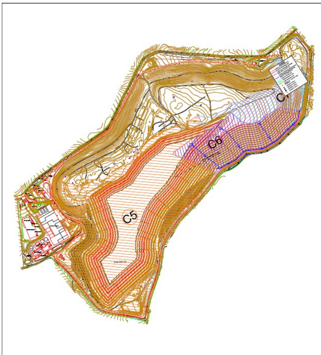
Figura Actualización de cuencas afectadas por el recredido. Cuencas C5, C6 y C7
