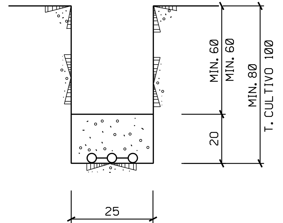
TRITUBO HORMIGONADO COTAS EN cm.
