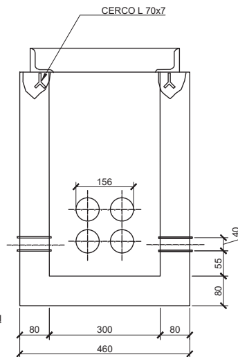
SECCIÓN B-B'
