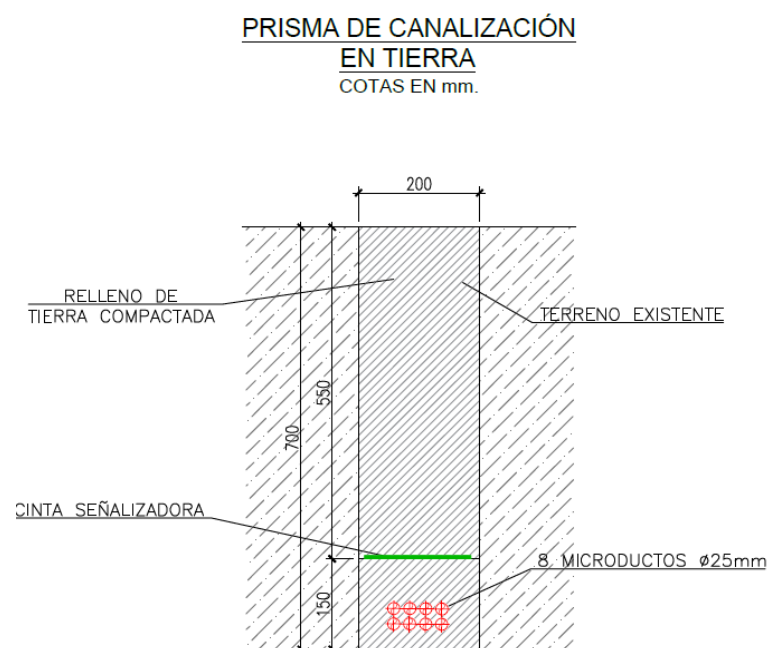
Figura 11: Prisma de canalización
