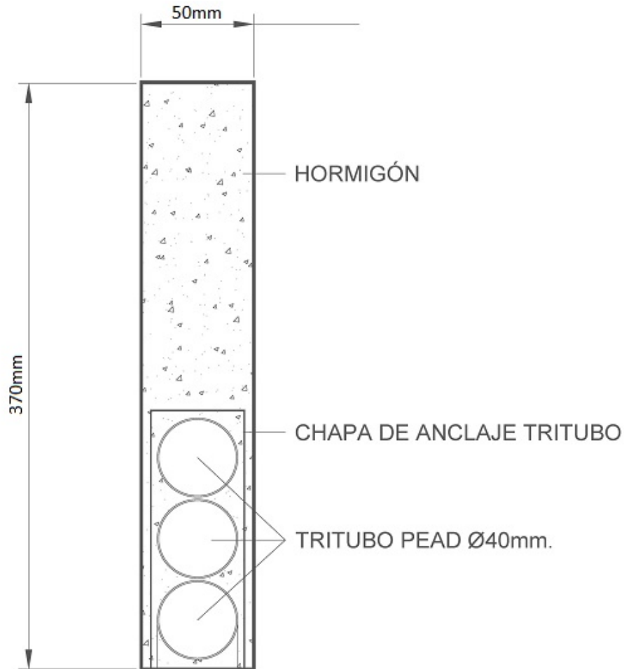
DETALLE CANALIZACIÓN H 1Tr 40 B1
