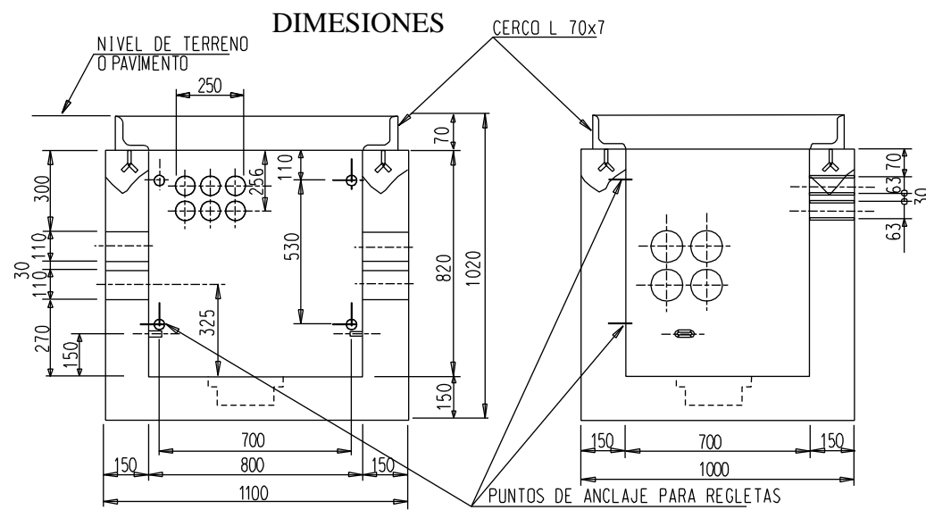
SECCIÓN B-B
