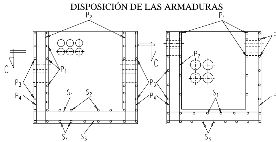
SECCIÓN B-B
