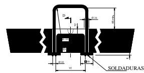
SECCIÓN B - B
