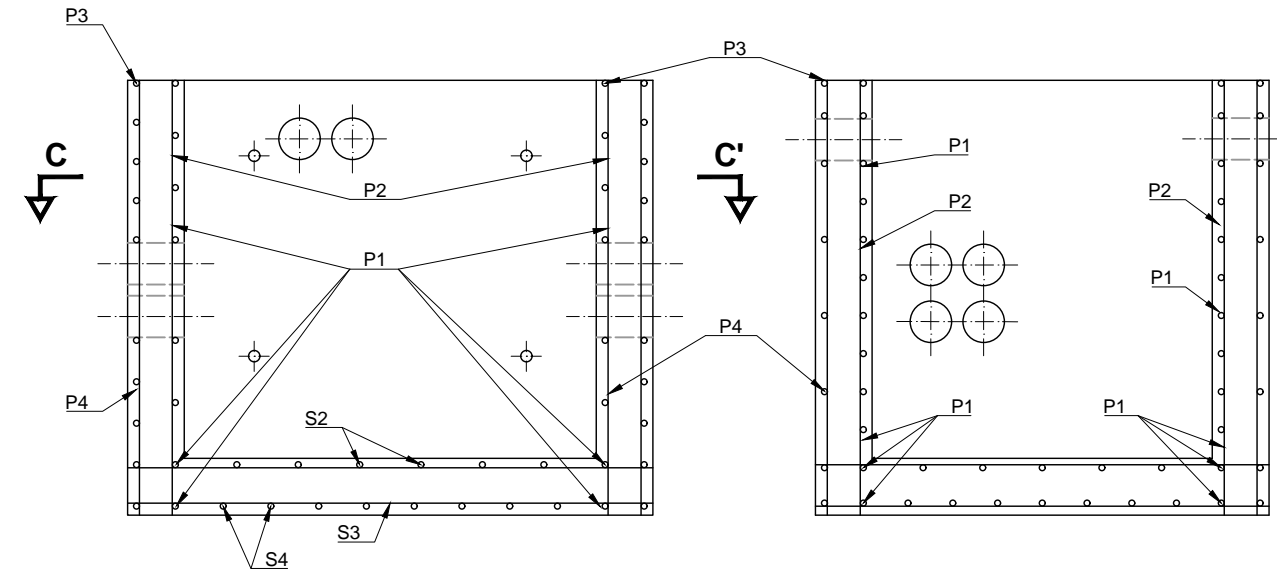
SECCIÓN A-A'
