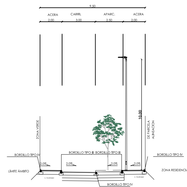
SECCIÓN VIARIO SUR DESDE BORDE VARIANTE A CALLE TENERÍA
