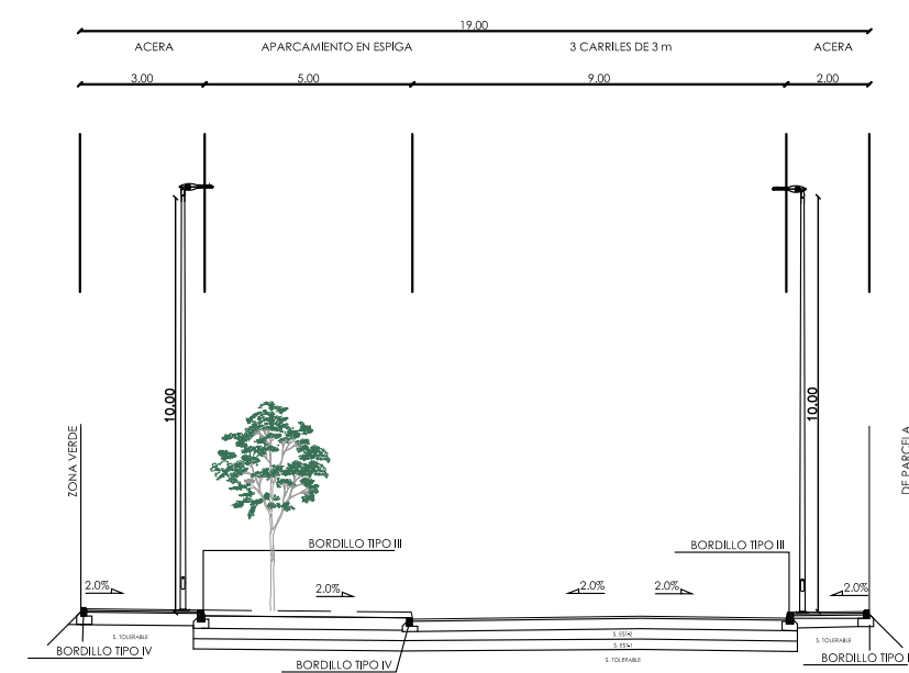
SECCIÓN VIARIO ANCHO JUNTO A VARIANTE
