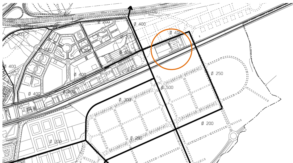
Fig. 6 Plano de distribución de agua de la RPGOU 01
