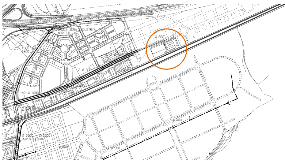
Fig. 7 Plano de la red de saneamiento de la RPGOU 01
