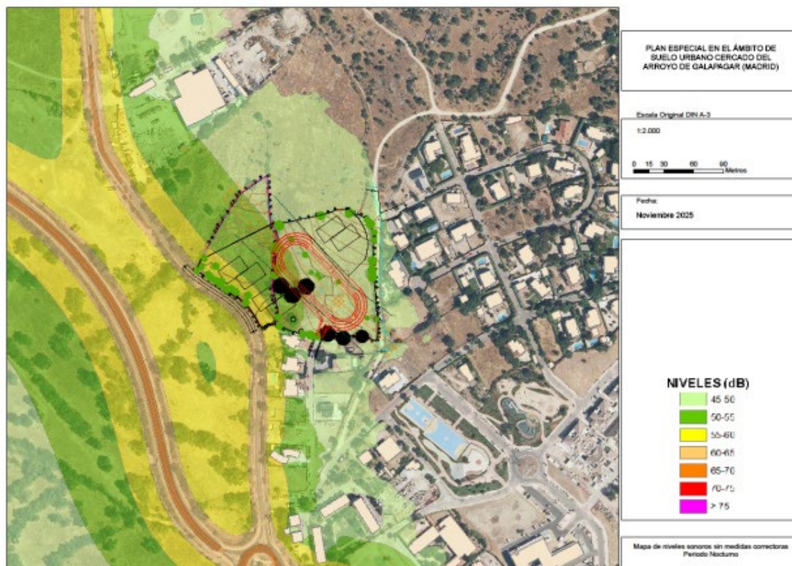
Figura 12. Mapa de niveles acústicos sin medidas correctoras periodo nocturno
