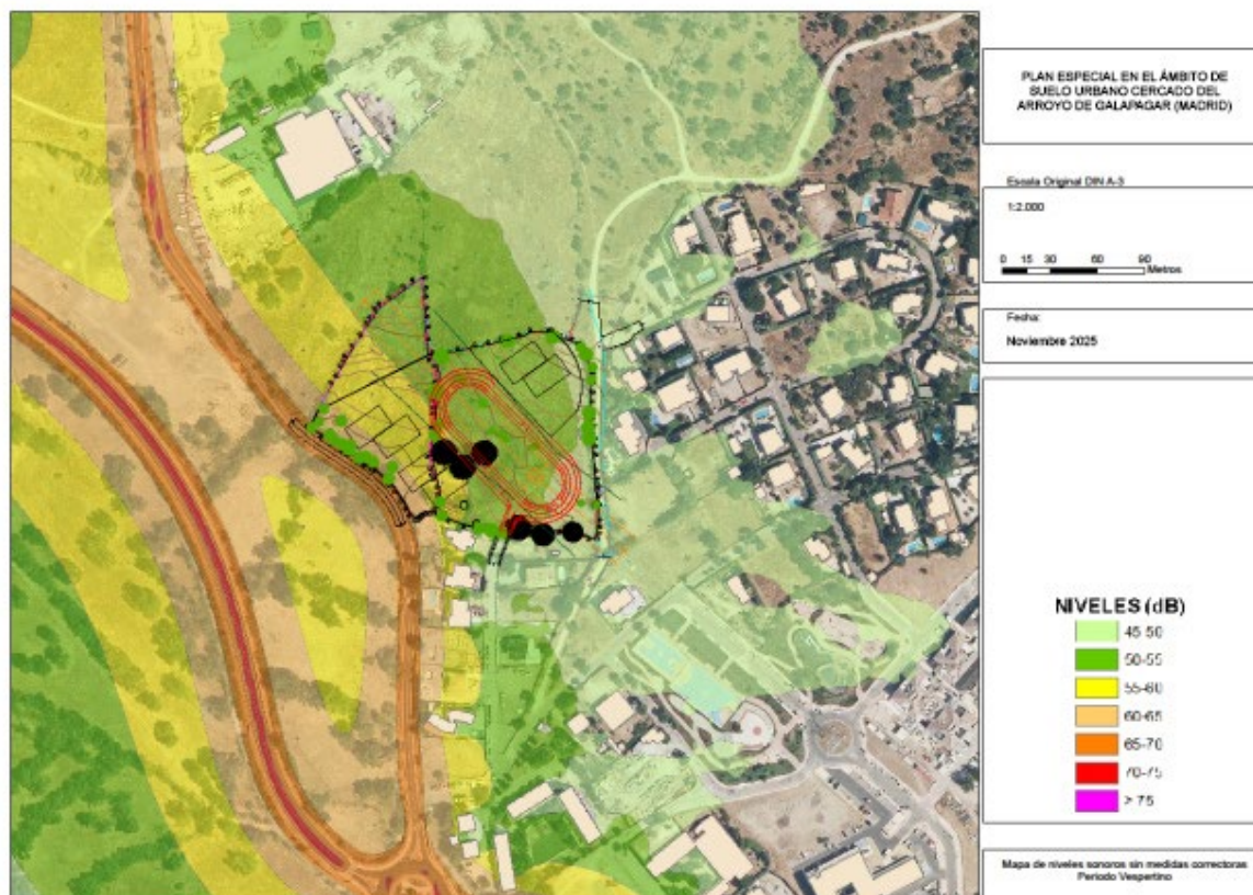
Figura 11. Mapa de niveles acústicos sin medidas correctoras periodo vespertino
