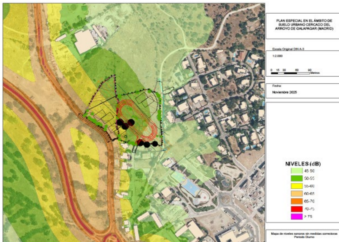
Figura 10. Mapa de niveles acústicos sin medidas correctoras periodo diurno
