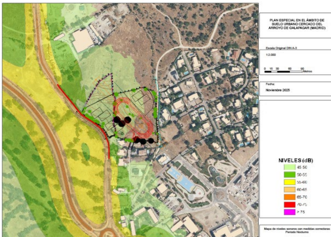
Figura 15. Mapa de niveles acústicos con medidas correctoras periodo nocturno
