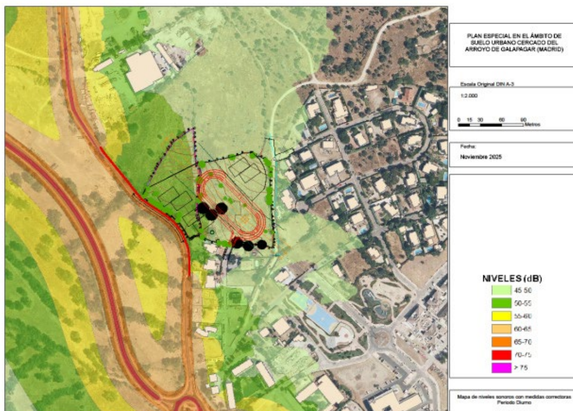
Figura 13. Mapa de niveles acústicos con medidas correctoras periodo diurno
