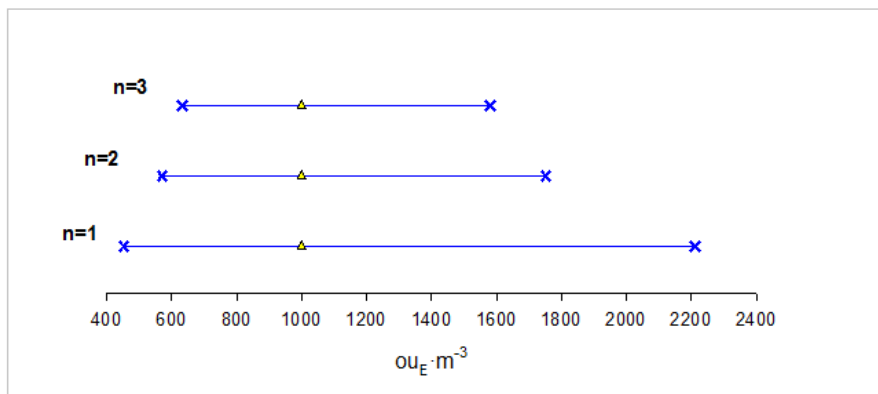
Figura 1. Relación entre el número de réplicas (n) y la incertidumbre cuando se analiza una muestra con una concentración real de 1.000 ouE·m -3 según los criterios exigidos por la norma EN13725
