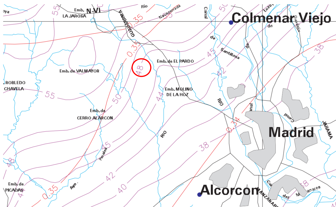
Figura 4. Mapa de isóneas de valor medio de la máxima precipitación diaria y coeficiente de variación de la zona de estudio. Fuente: Máximas Lluvias Diarias en la España Peninsular, CEDEX
