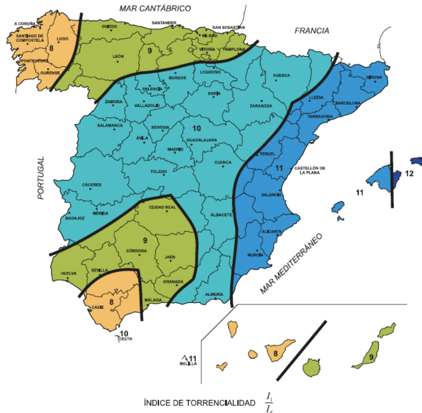
Figura 5. Mapa del índice de torrencialidad ( I_1/I_a ). Fuente: Norma 5.2-IC
