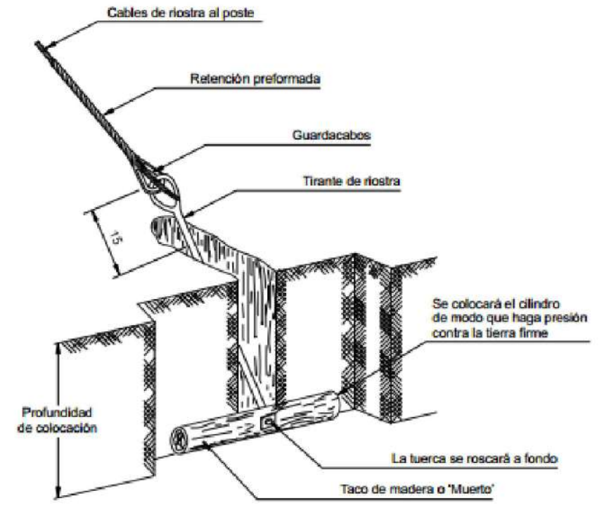
TIRANTES DE RIOSTRAS TIPOS A Y B
