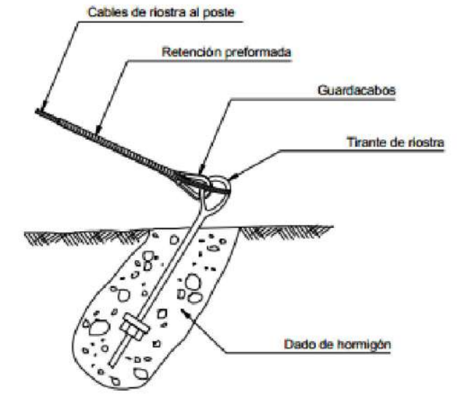
TIRANTE DE RIOSTRA TIPOS C
