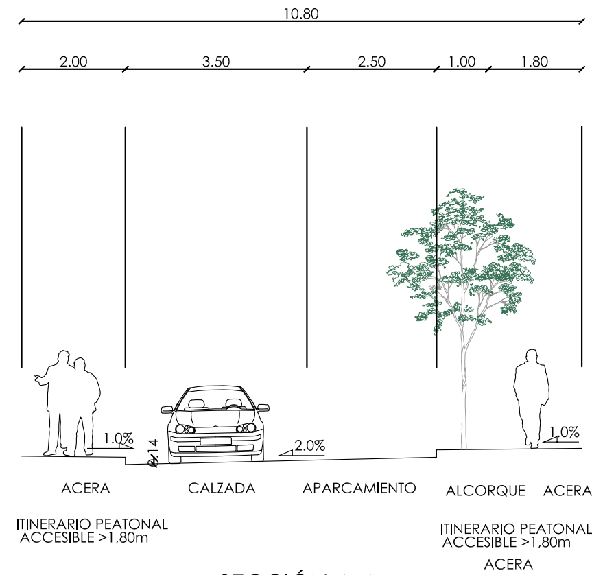
SECCIÓN A-A
