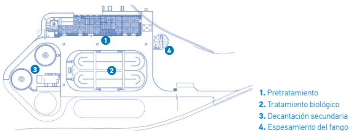
Figura 116. Esquema EDAR de Ambite (fuente: Canal de Isabel II)
