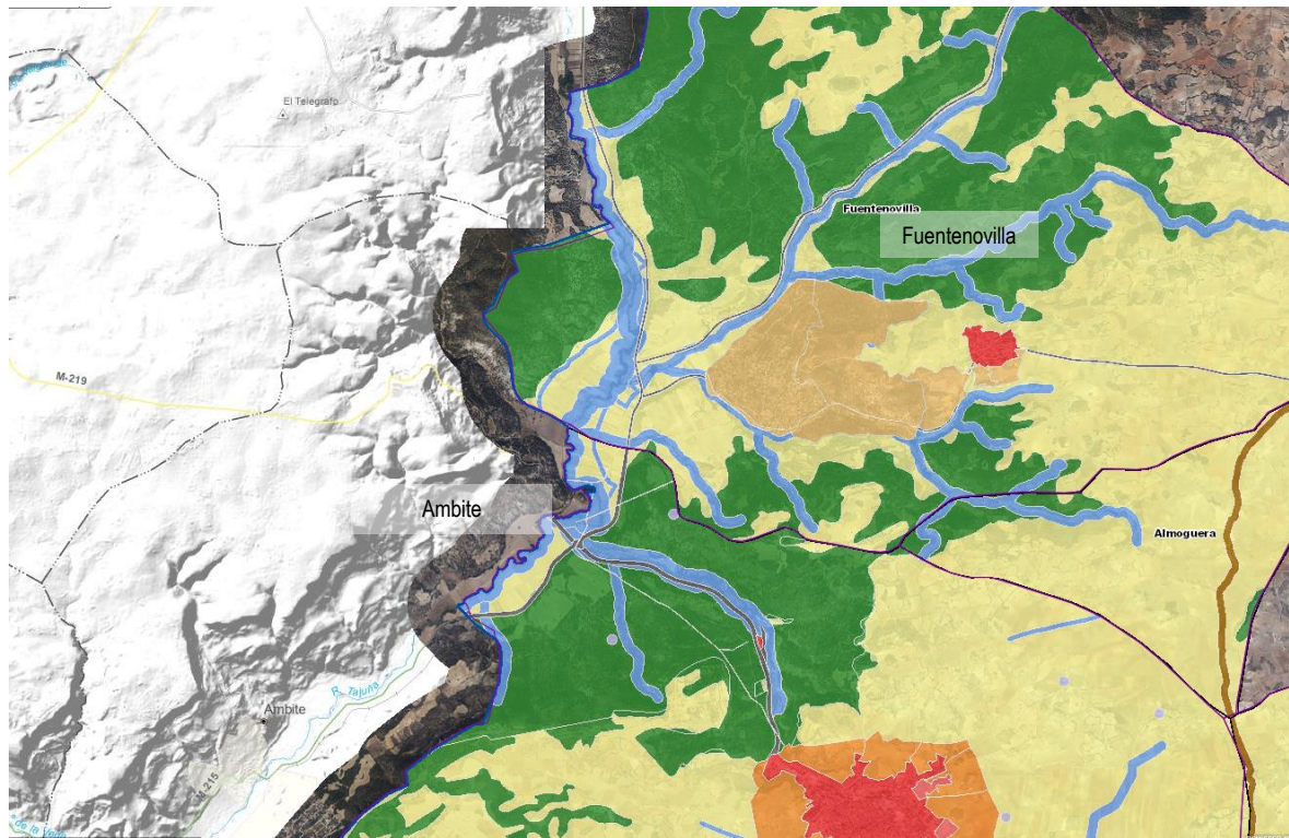
Figura 151. Plano de Clasificación de Suelo de Fuentenovilla. Sistema de Información Territorial de la Comunidad de Castilla La Mancha.
