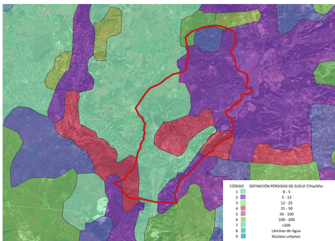
Figura 16. Mapa de Estados Erosivos (fuente: MITECO).
