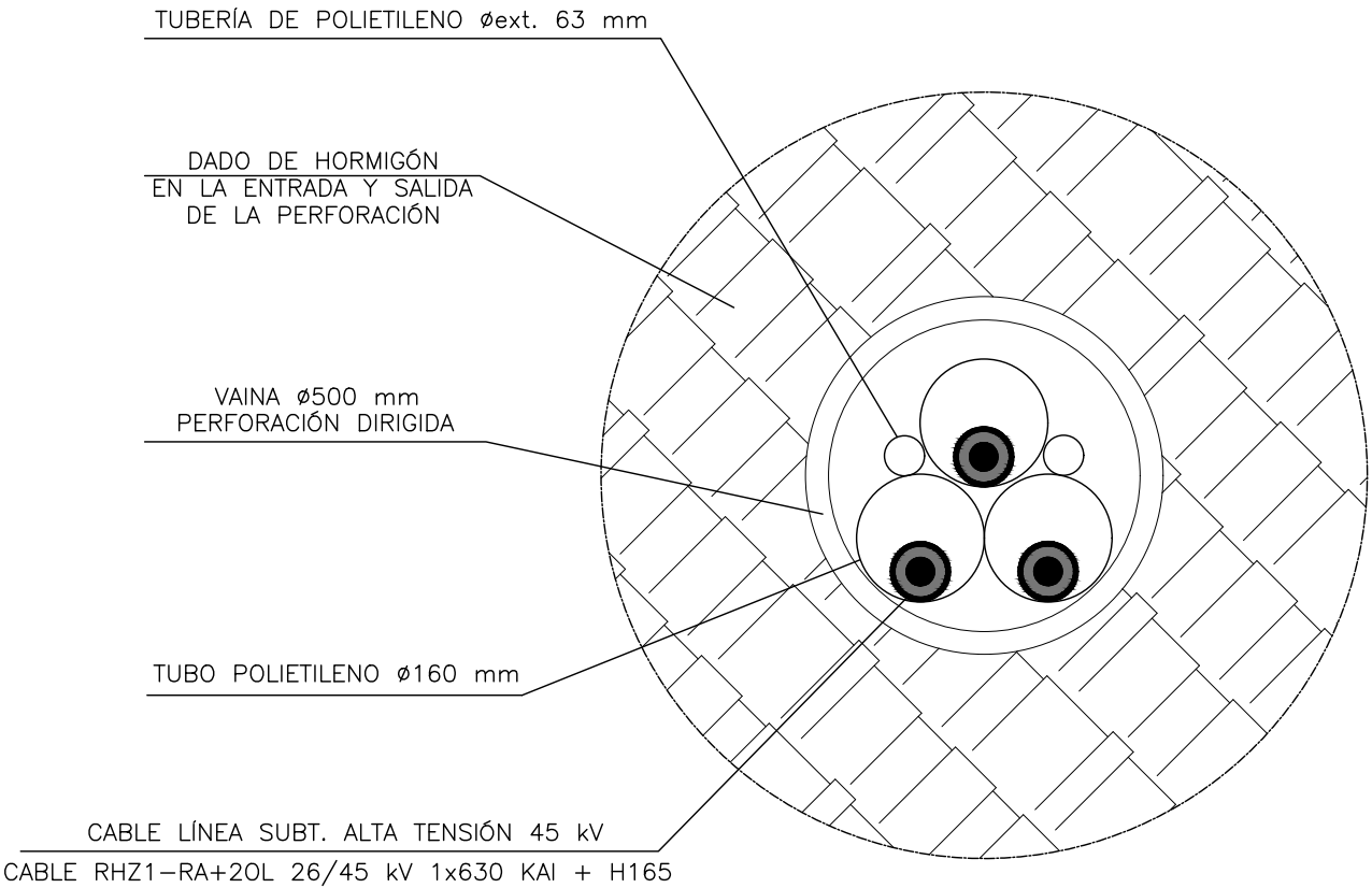
DETALLE VAINA Escala 1: 10
