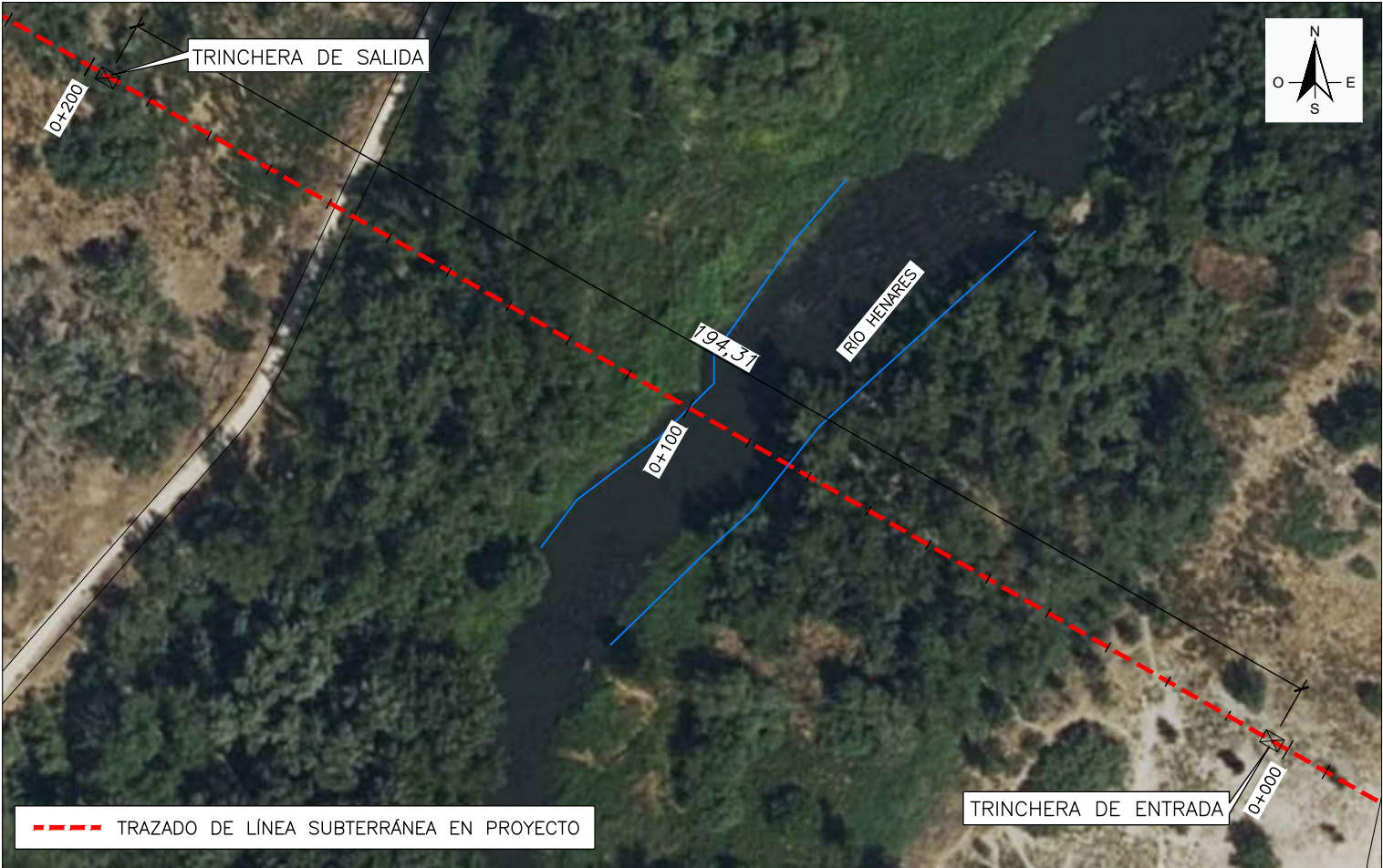
PLANTA CRUZAMIENTO CON RÍO HENARES Escala 1:1.000
