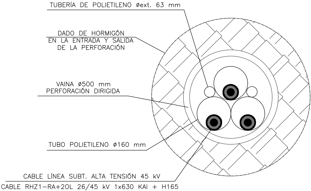
DETALLE VAINA Escala 1: 10
