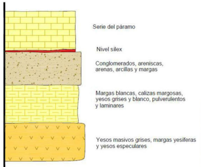
Figura 5.3.- PI Bruselas. Columna estratigráfica tipo.
