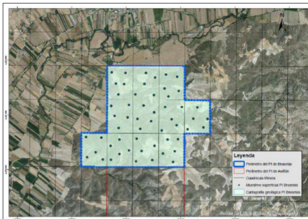
Figura 8.4.- Muestreo y cartografía geológica en el PI de Bruselas.
