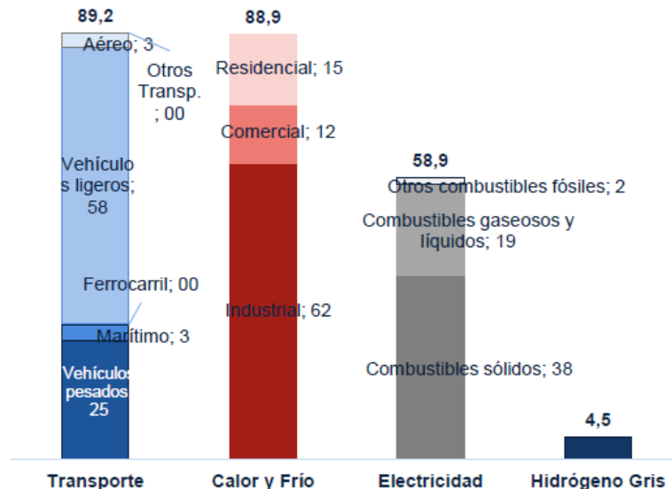
Emisiones CO2 de uso energético por sector, España 2018 MT CO2 (1)
