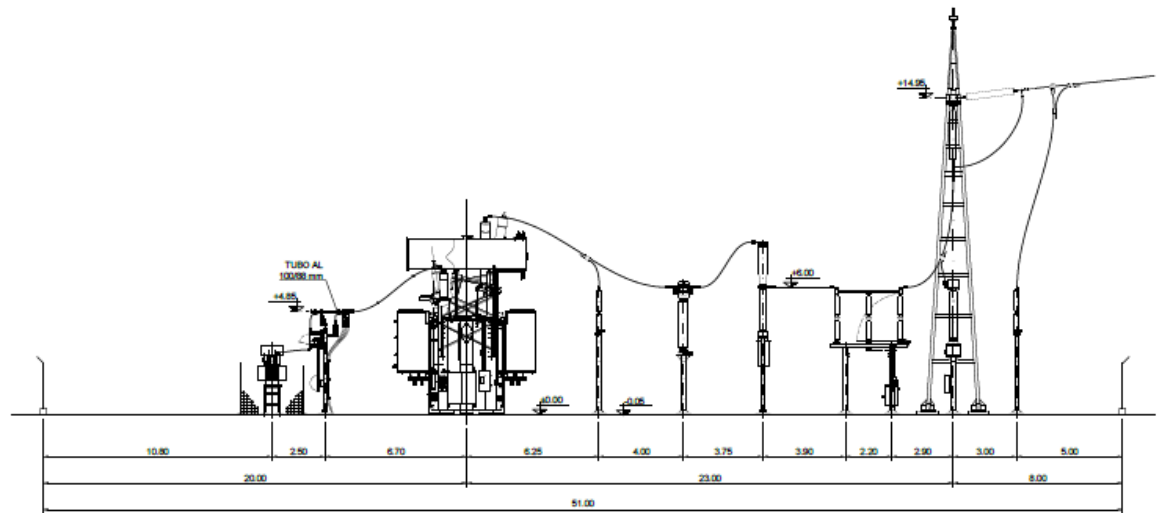
SECCION A-A
