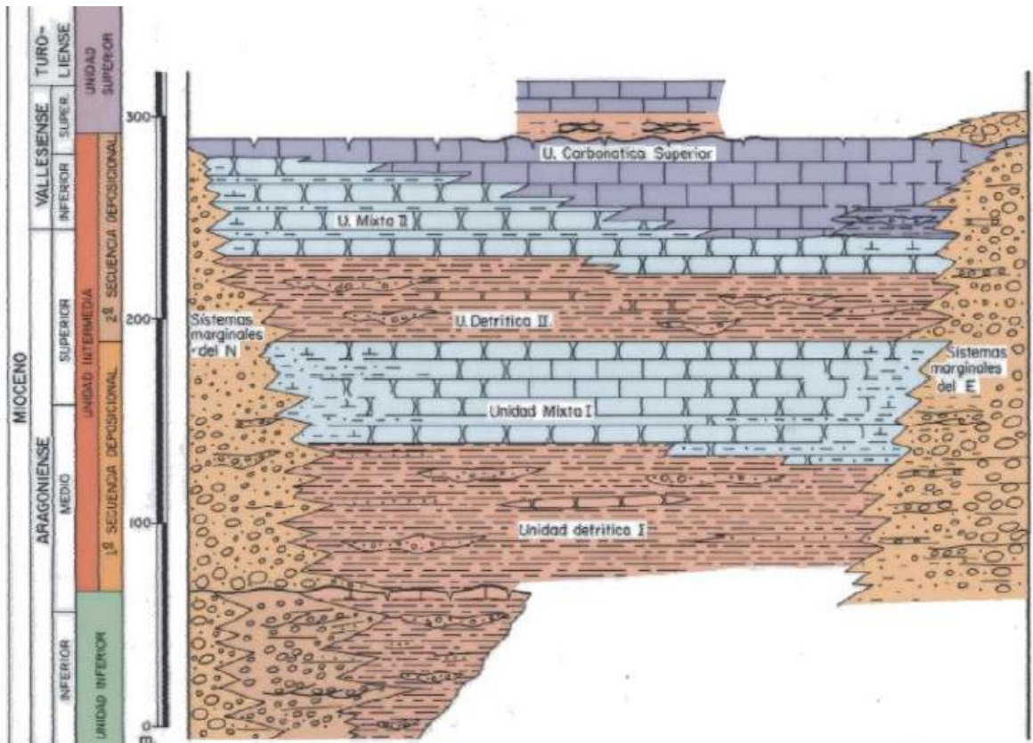
Sucesión estratigráfica de la Cuenca de Madrid
