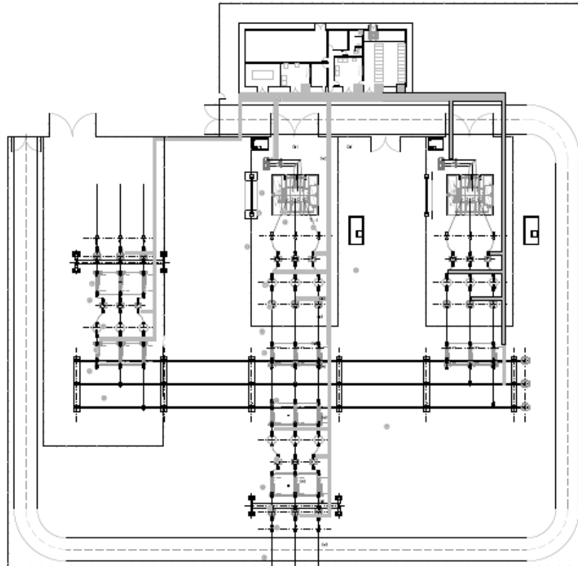
Planta de la SET Aldehuela (Fuente: Proyecto de la SET Aldehuela realizado por dos grados )
