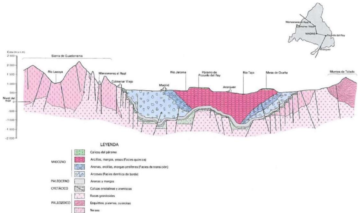
Corte simplificado de la Depresión del Tajo (ITGE, 1989)
