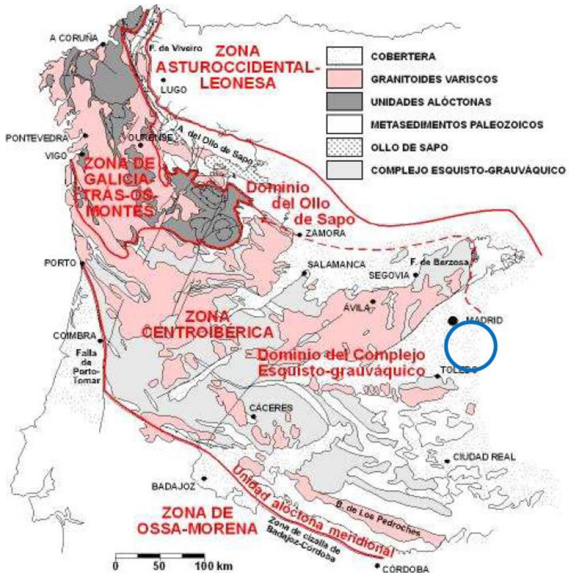
Subdivisión en dominios de la Zona Centro Ibérica, según Martínez Catalán et al. (2004). Geología de España. IGME.
