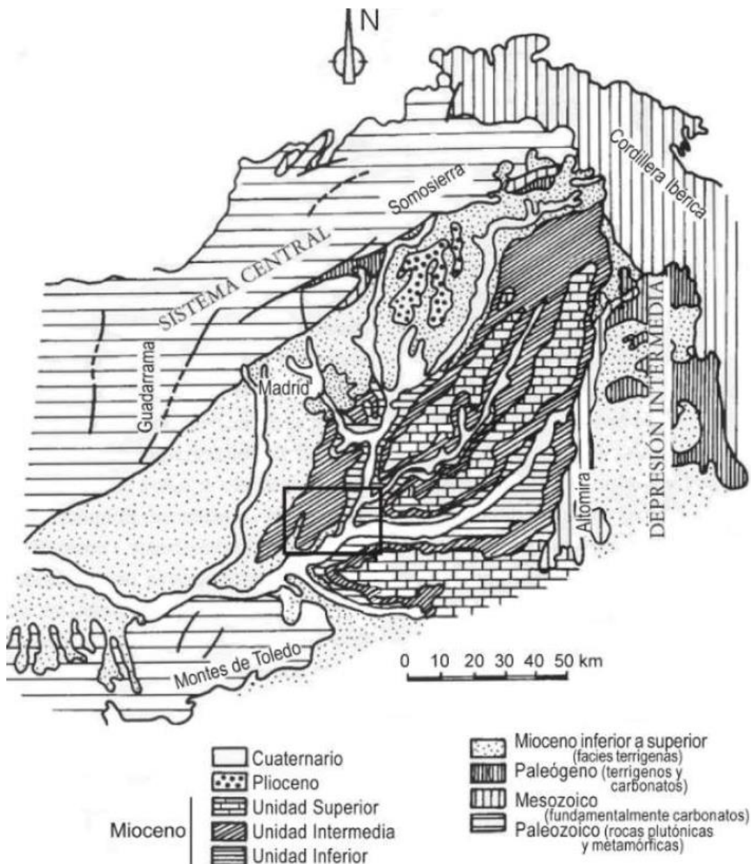
Esquema estratigráfico de la Depresión del Tajo
