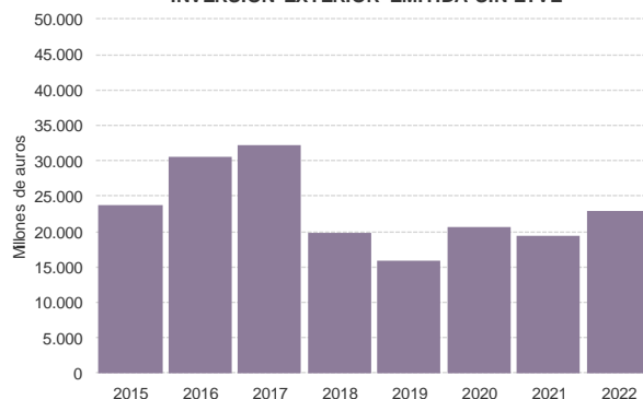
COMUNIDAD DE MADRID INVERSIÓN EXTERIOR EMITIDA SIN ETVE
