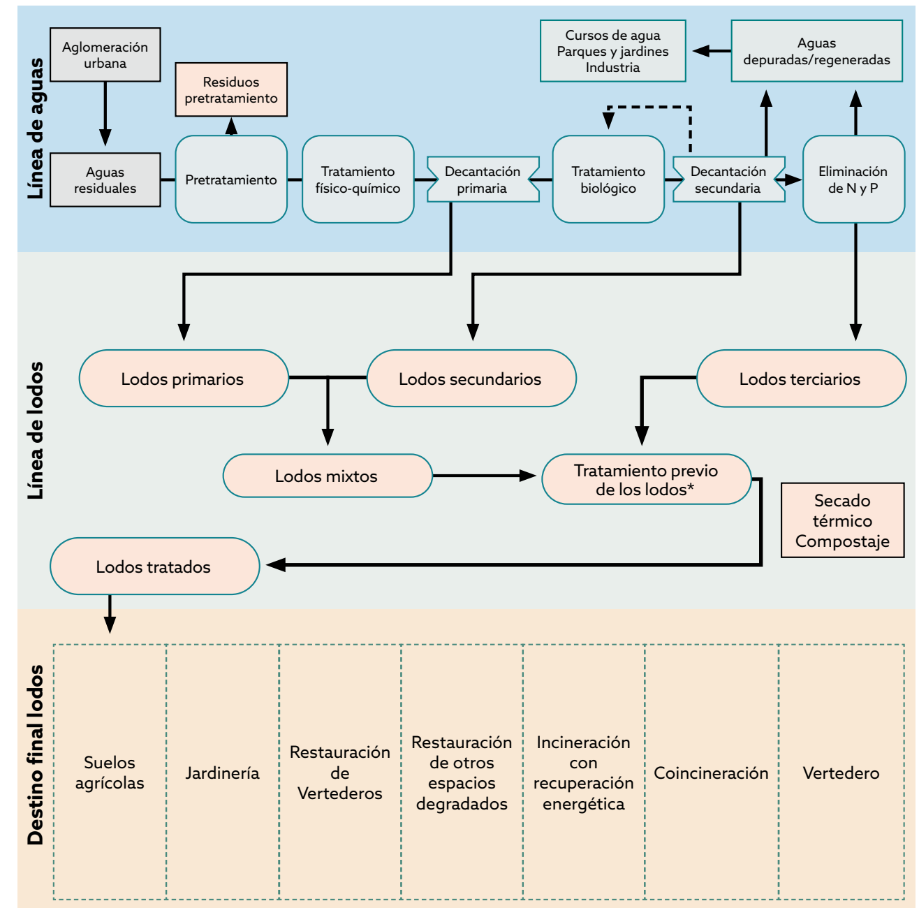
Figura 18-1. Proceso de gestión de los lodos de la depuración de las aguas residuales.
