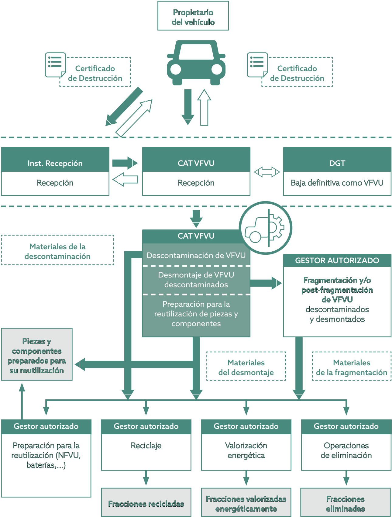
Figura 15-1. Modelo de gestión de vehículos al final de su vida útil.
