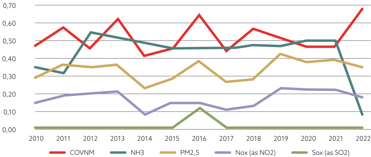
Gráfico 2-6. Evolución de los contaminantes atmosféricos (kt) en el sector de tratamiento y eliminación de residuos en la Comunidad de Madrid.
