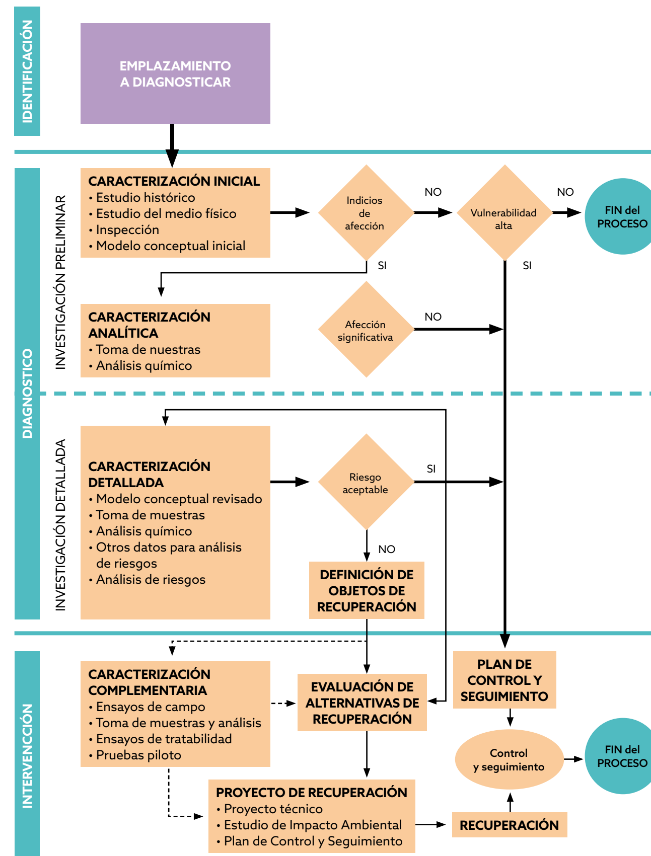
Figura 20-1. Diagrama del modelo de gestión de suelos contaminados.
