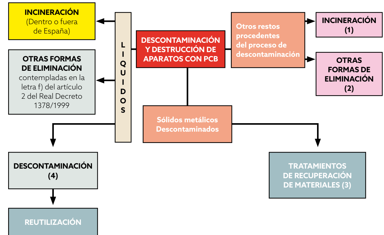
Figura 17-1. Diagrama del proceso para la descontaminación y destrucción de aparatos con PCB.
