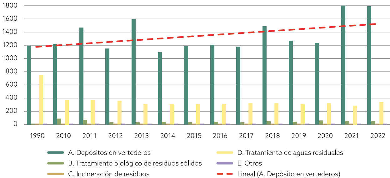
Gráfico 2-5. Evolución de las emisiones de GEI derivadas del tratamiento y eliminación de residuos (CO 2 equivalente - Kt), en la Comunidad de Madrid.
