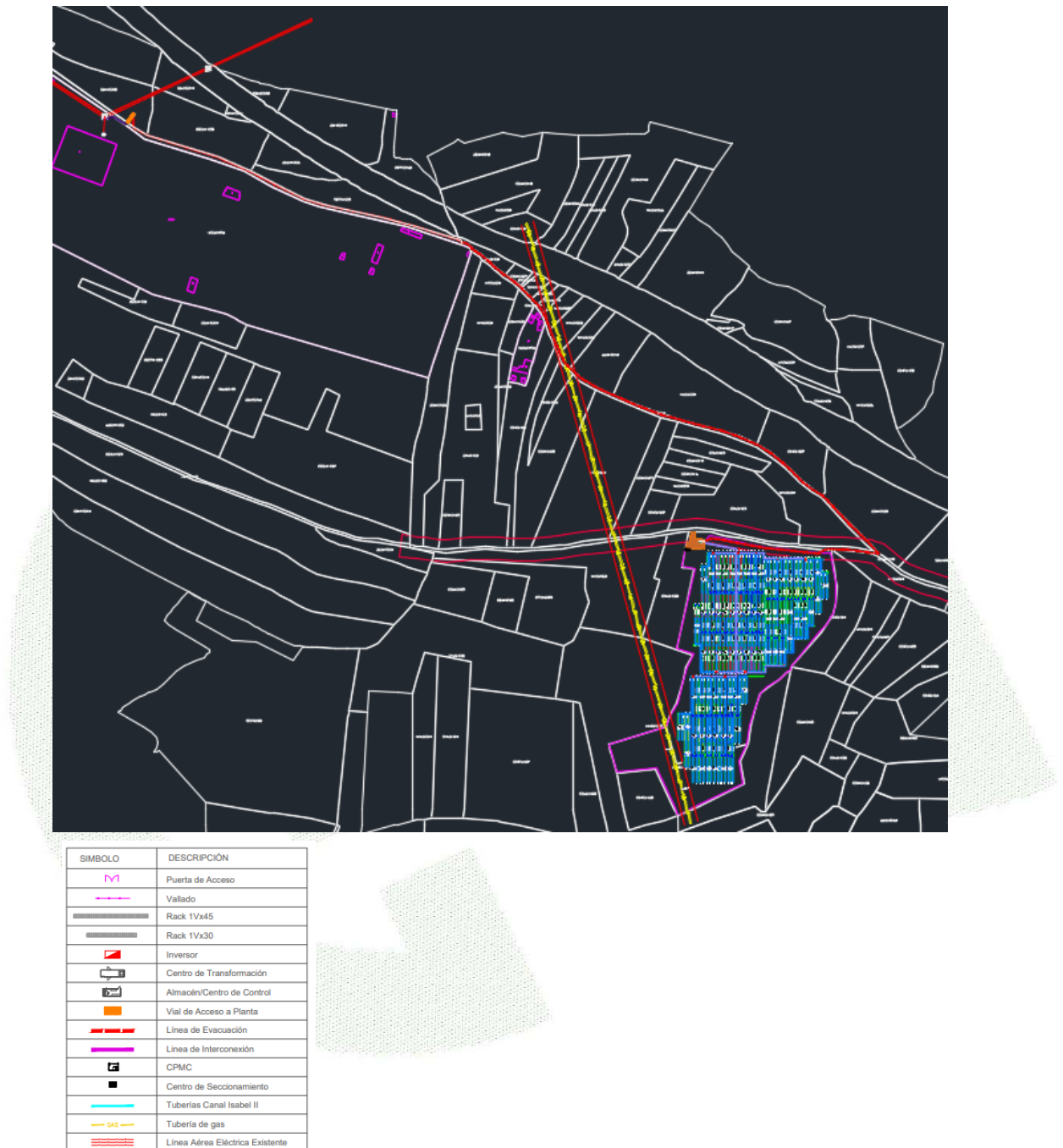
Figura 3: Instalación proyectada en las parcelas de estudio en Cobeña (Madrid).
