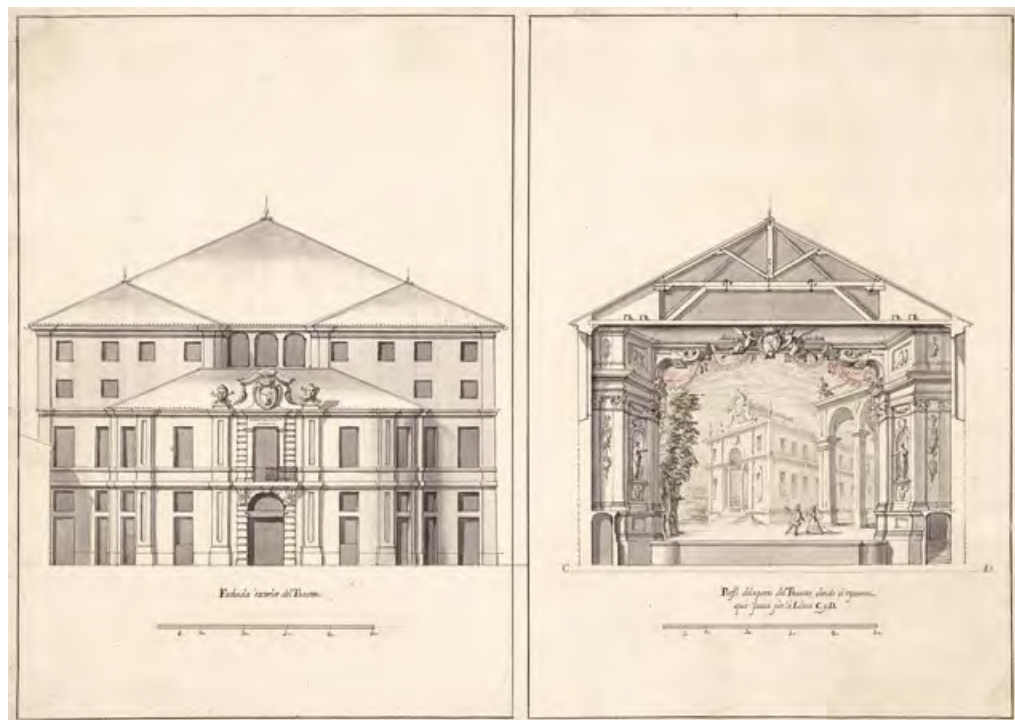
Proyecto para el Coliseo de la Cruz de Madrid. Fachada y Embocadura. Tinta sobre papel verjurado Archivo de Villa (Madrid), sig. o,69-23-3
