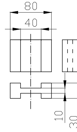
DETALLE LLAVE
