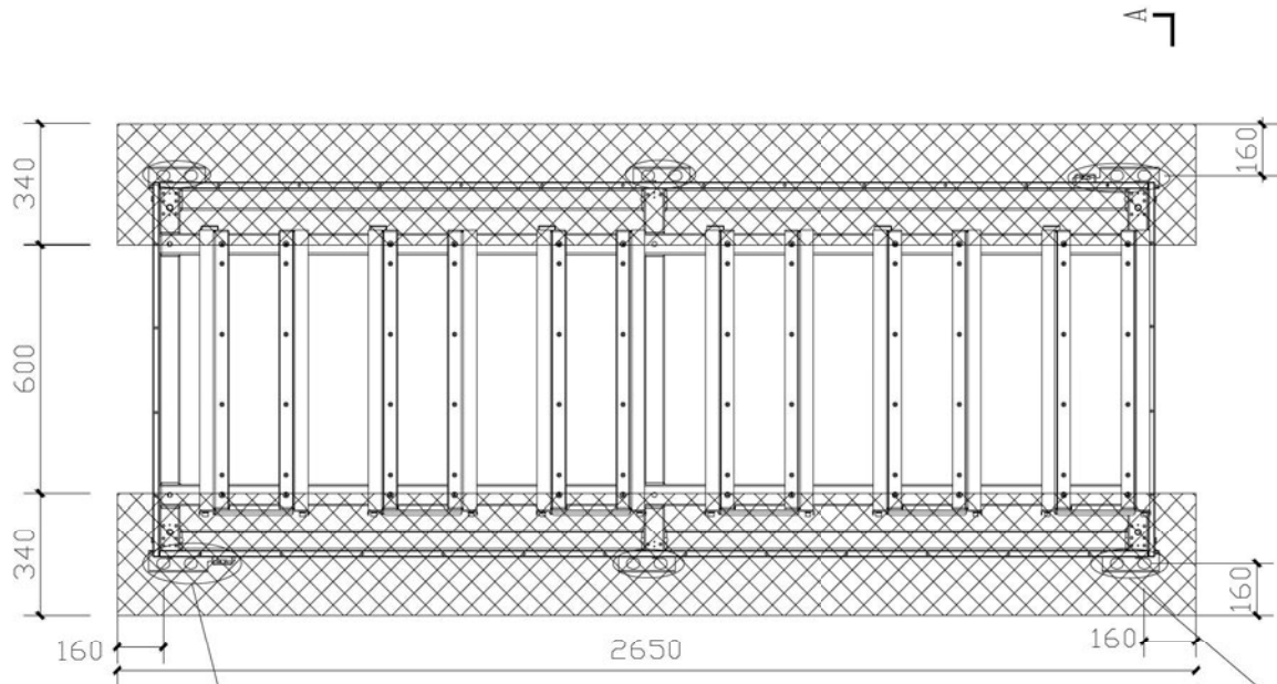
Plano Cimentación
