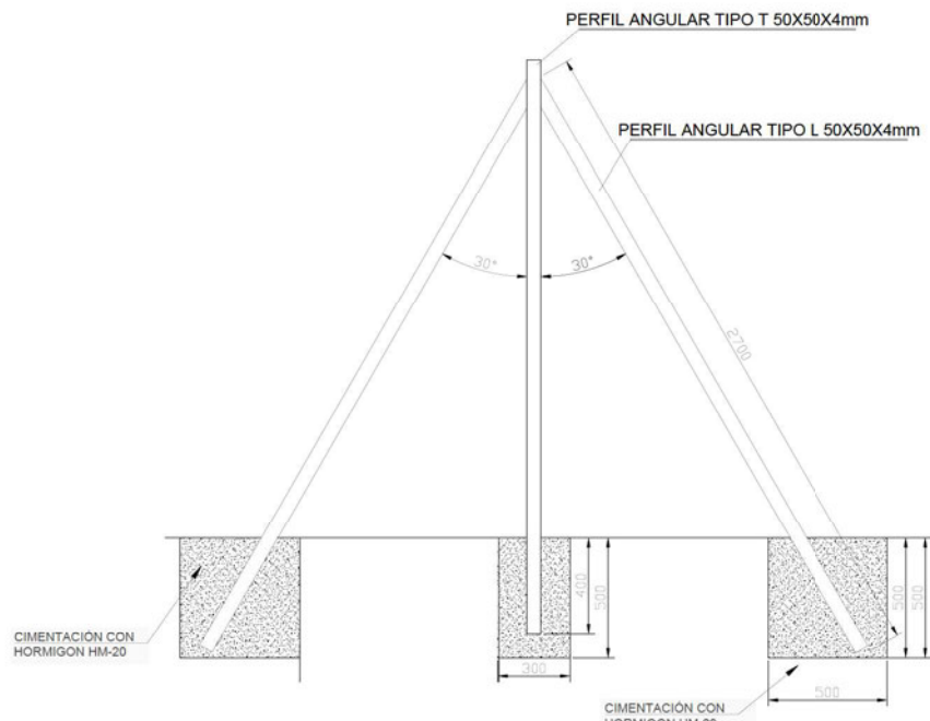
POSTE DE TENSION POSTE INTERMEDIO
