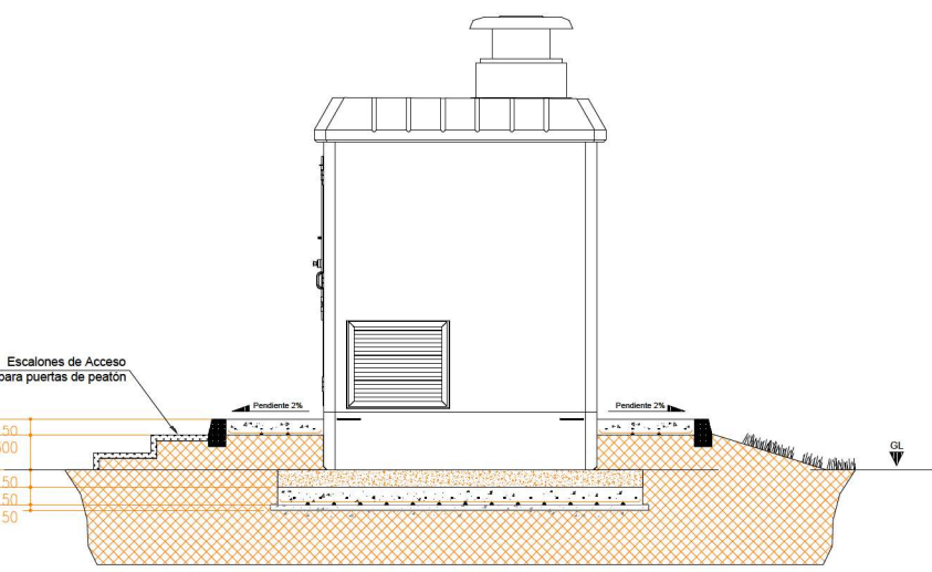
VISTA LATERAL DERECHA
