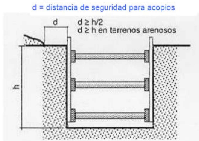
Figura 2. Distancia de seguridad entibaciones
