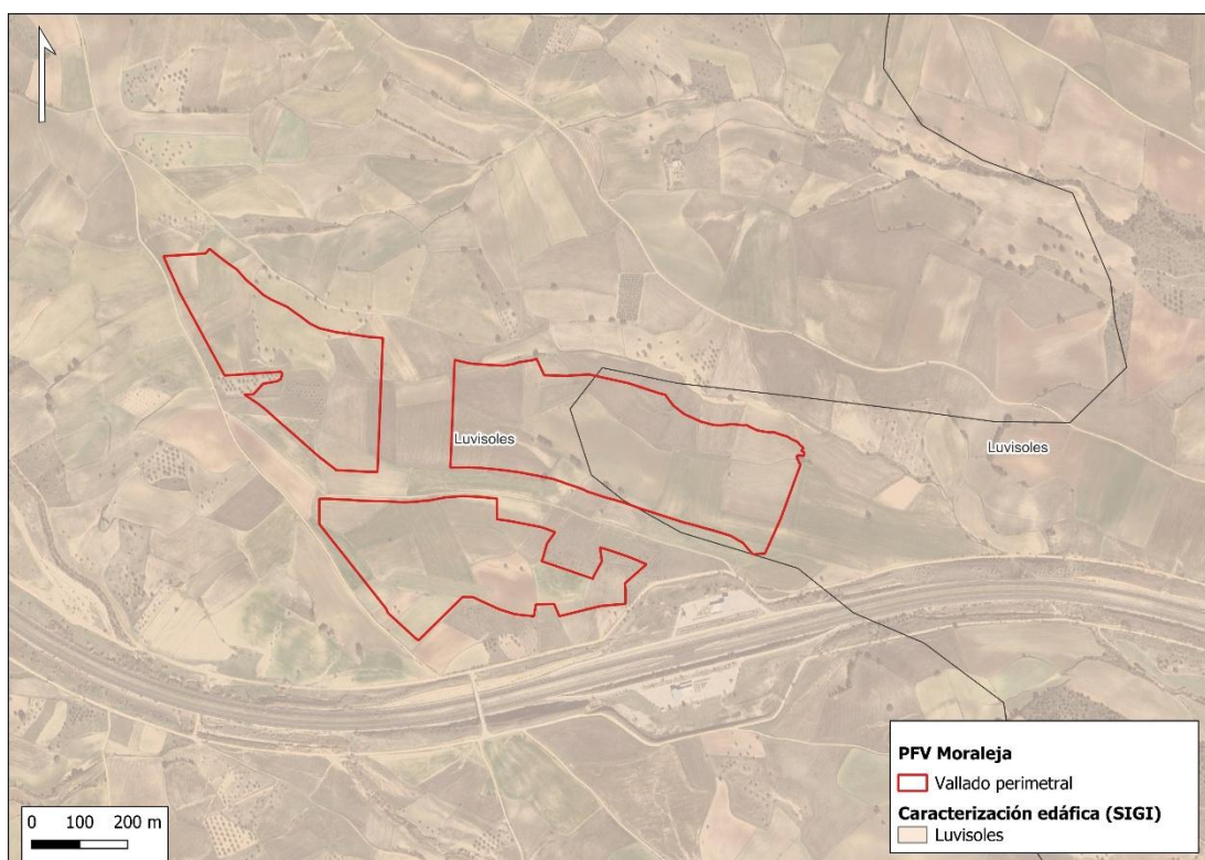
Figura 3. Tipo de suelo en el que se sitúa la implantación de la PSFV "Moraleja" (Fuente: elaboración propia a partir de la información de la FAO).
