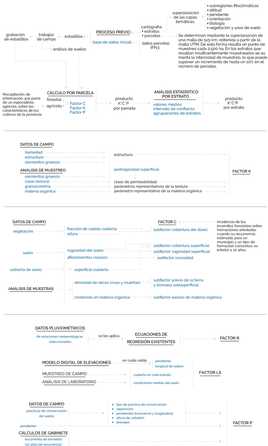
Figura 7. Mapa conceptual del cálculo de los niveles de pérdida de suelo por erosión laminar. Fuente: Resumen Nacional del INES 2022.
