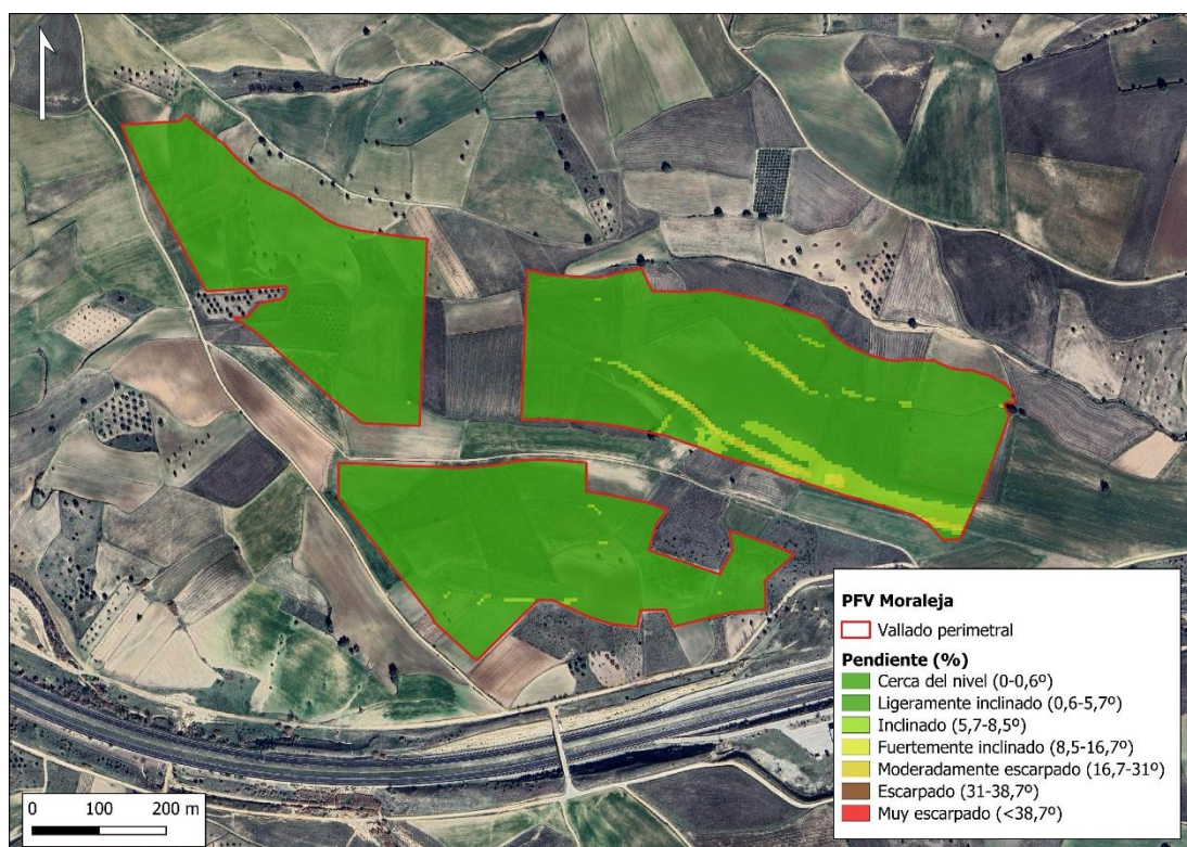
Figura 1. Pendientes correspondientes al área de implantación de la PSFV "Moraleja" (Fuente: elaboración propia a partir de la información CNIG).
