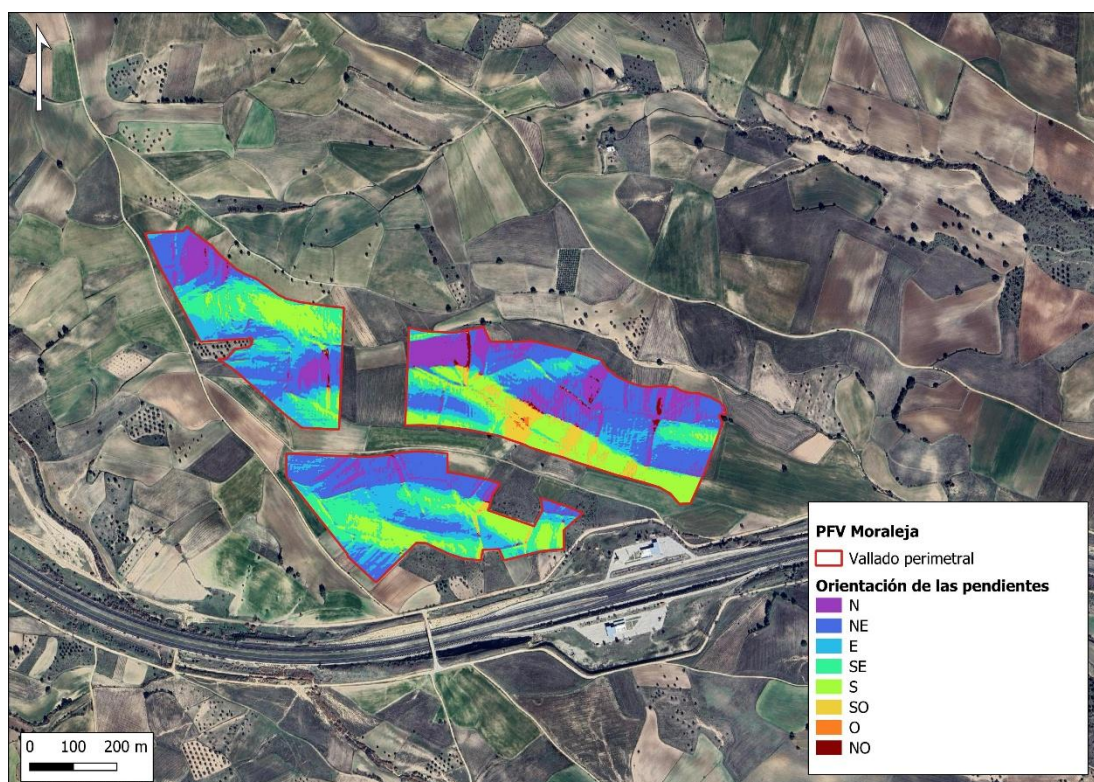
Figura 2. Orientación de las pendientes correspondientes al área de implantación de la PSFV "Moraleja" (Fuente: elaboración propia a partir de la información CNIG).
