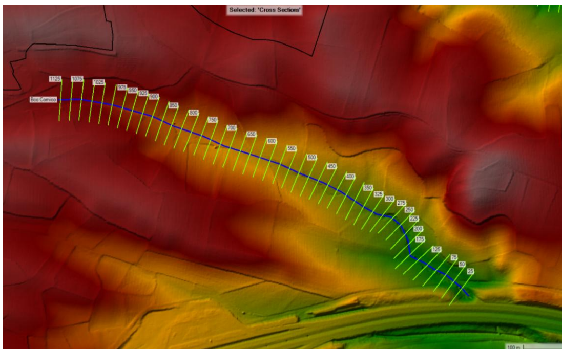
Figura 3. Secciones transversales consideradas en el modelo HEC-RAS, para el Barranco del Cómic.
