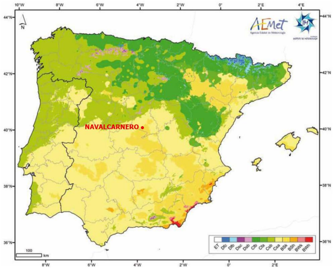
Figura 11. Mapa de España. Clasificación de Köppen-Geiger
