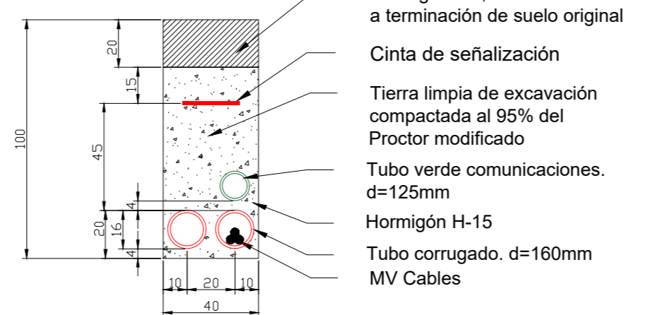
TRAMO ZANJA LÍNEA DE EVACUACIÓN SIN CRUZAMIENTO
