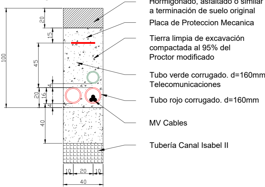
TRAMO ZANJA LÍNEA DE EVACUACIÓN CRUZAMIENTO CANAL ISABEL II
