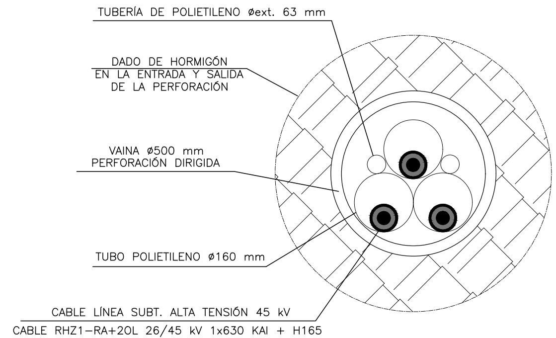
DETALLE VAINA Escala 1: 10
