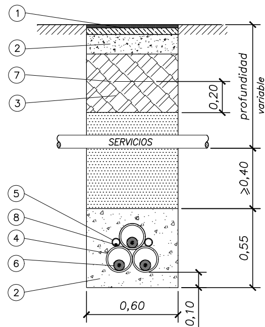
SECCIÓN TIPO CRUZAMIENTO CON SERVICIOS CANALIZACIONES DE GAS
