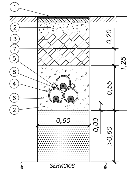
SECCIÓN TIPO CRUZAMIENTO CON SERVICIOS CANALIZACIONES OLEODUCTO
