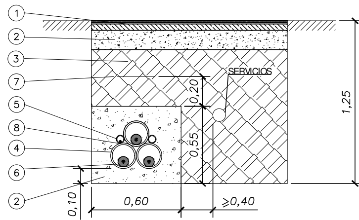
SECCIÓN TIPO PARALELISMO CON SERVICIOS CANALIZACIONES DE GAS
