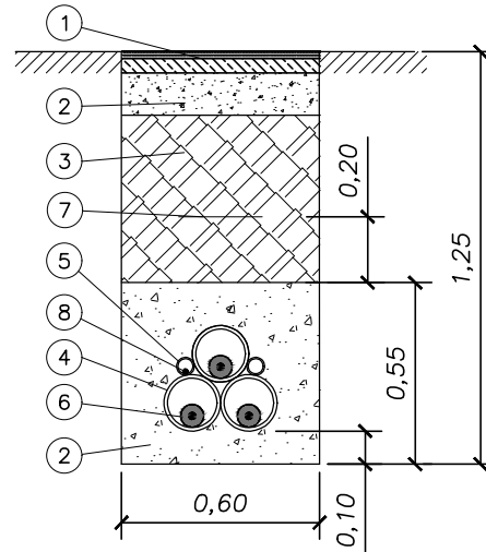
ZANJA PARA UN CIRCUITO ALTA TENSIÓN EN ZONA DE CALZADA O ACERA
