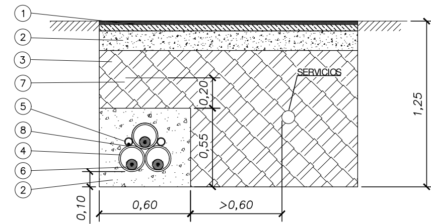
SECCIÓN TIPO PARALELISMO CON SERVICIOS CANALIZACIONES OLEODUCTO
