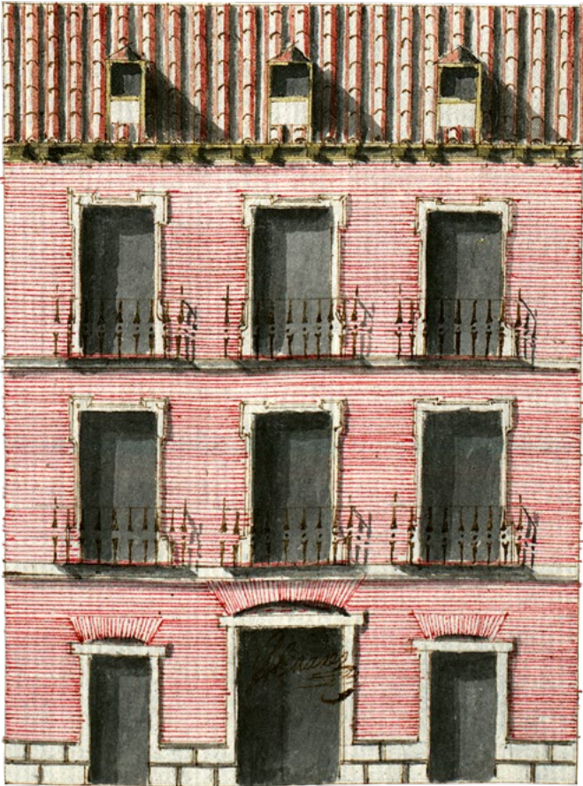
1738. Alzado de una casa ubicada en la calle de Carretas, incluido en la escritura para demoler dicha propiedad y volverla a reedificar según figura en el diseño. AHPM. DG.85
